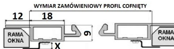
Rys. 1 Wymiarowanie standardowe
