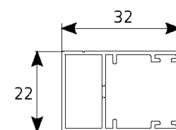
Prowadnica prosta
