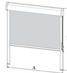
Rys.3 Szerokość i wysokość całkowita rolety
