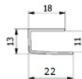
Rys 4 Prowadnica przestrzenna
