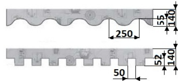
Rys. 2 Falbana typ 1
