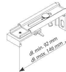
Rys. 2 Montaż do ściany – wieszak B
