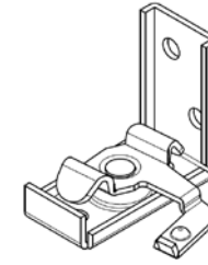
Rys. 3 Mocowanie rynny górnej
