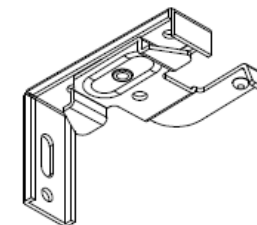
Rys. 3 Mocowanie rynny górnej - uchwyt Twist na wieszaku kątowym
