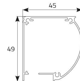
Przekrój skrzynki
