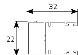
Prowadnica prosta
