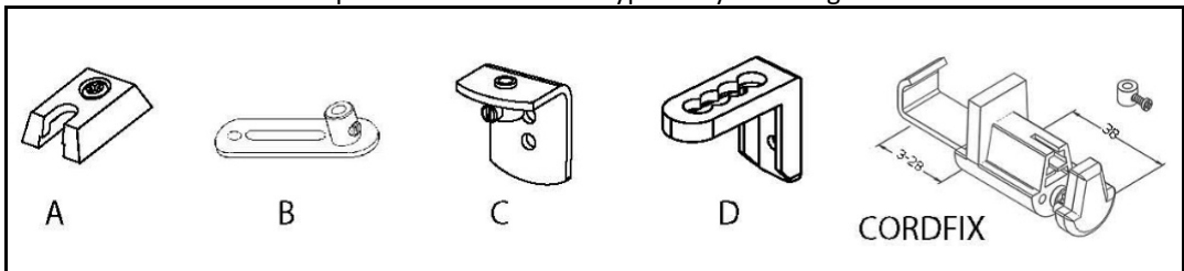
przewodzenie boczne - typ uchwytu dolnego
