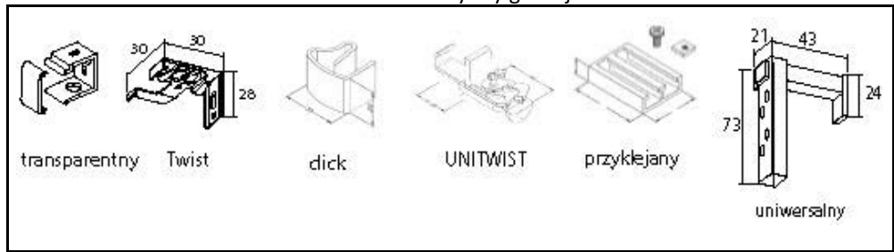
mocowanie rynny górnej
